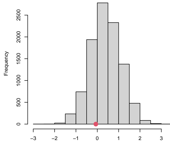
Posterior at time t=20
