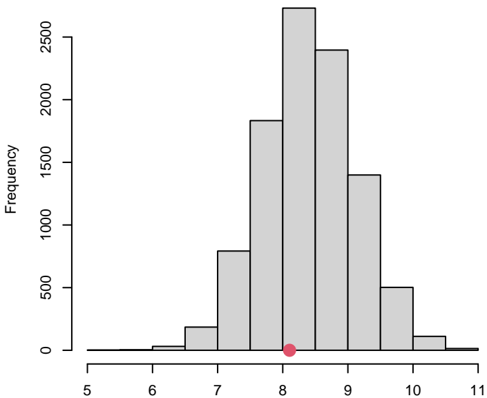
Posterior at time t=60
