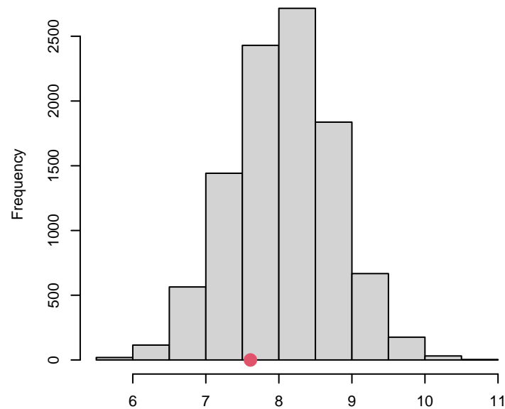
Posterior at time t=80
