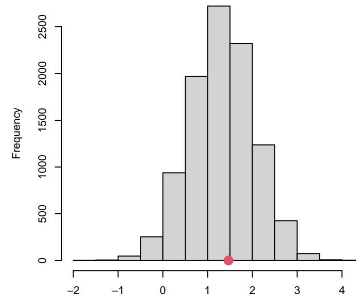
Posterior at time t=40
