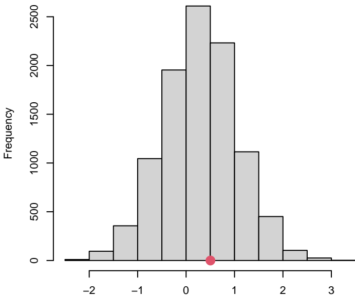
Posterior at time t=1
