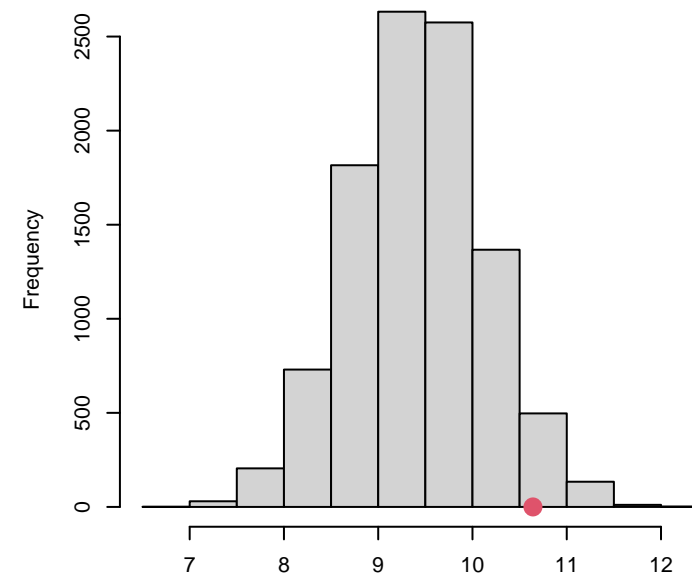
Posterior at time t=100
