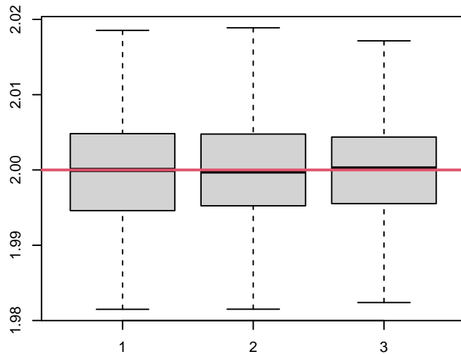
lasso
