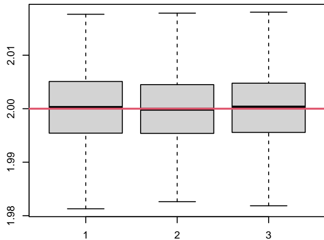
lasso
