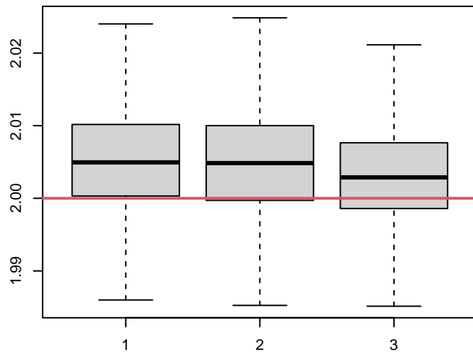
lasso
