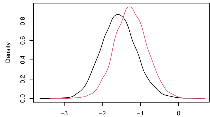
beta(62)
