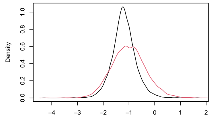
beta(100)
