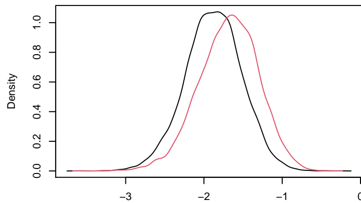
beta(50)
