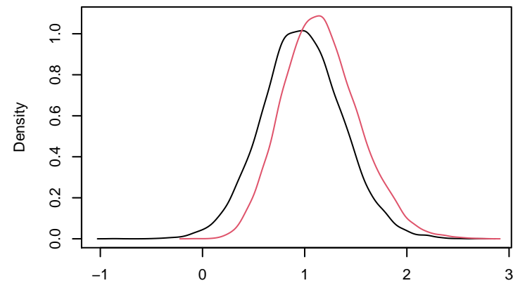
beta(25)
