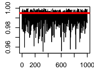
pi
