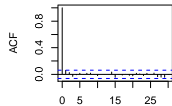
sig2
