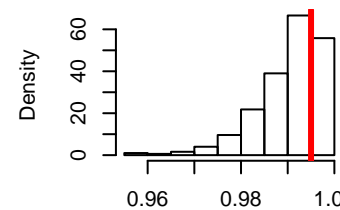
pi
