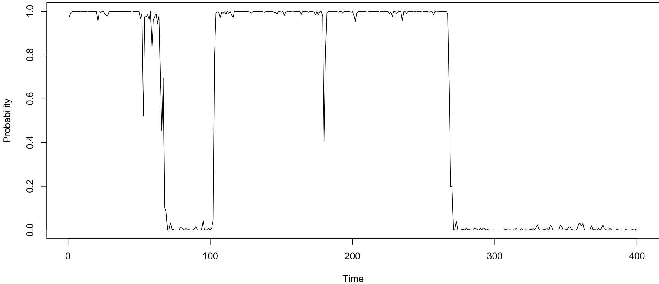
Prob(S(t)=1|D(t))
