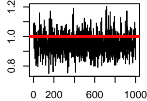
sig2
