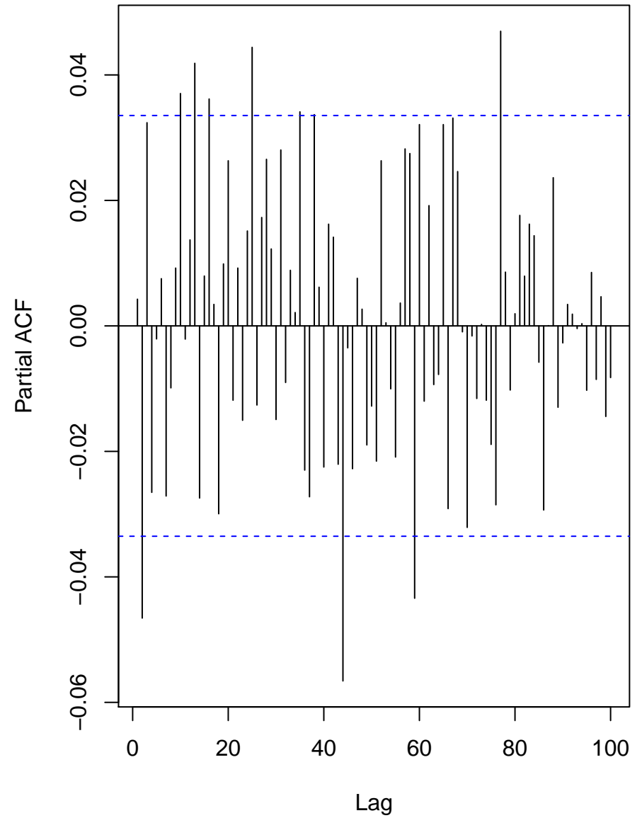
Log returns
