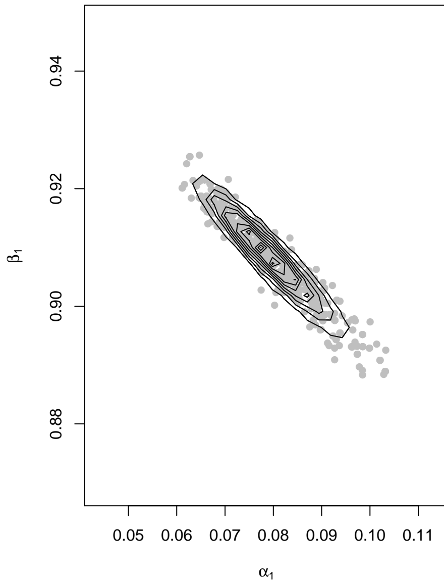
Posterior contours and draws
