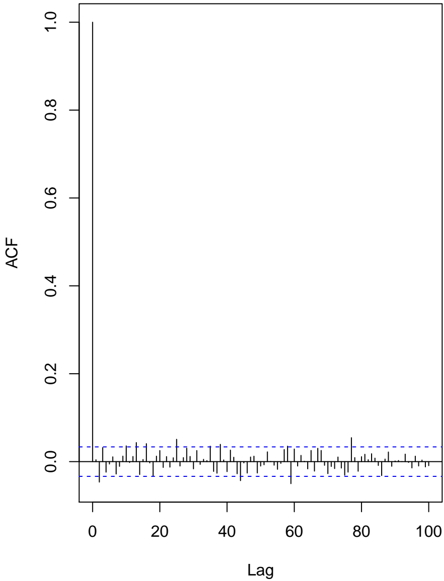
Log returns
