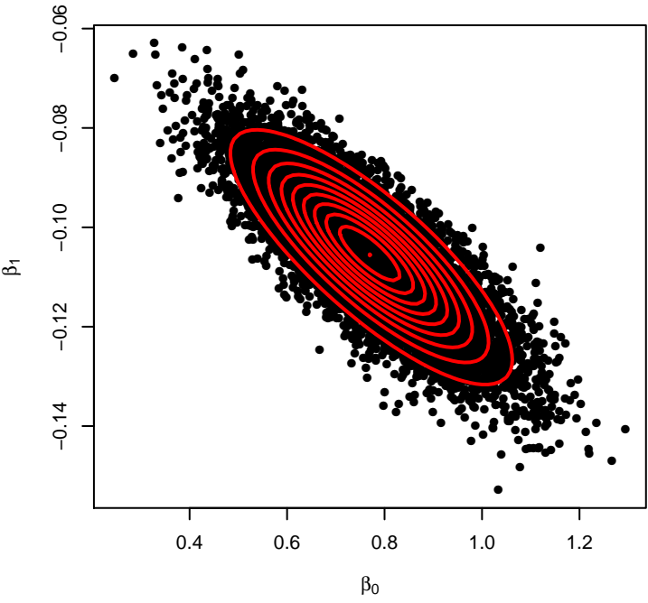
Posterior distribution
