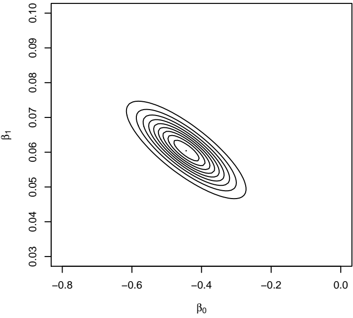
Posterior distribution
