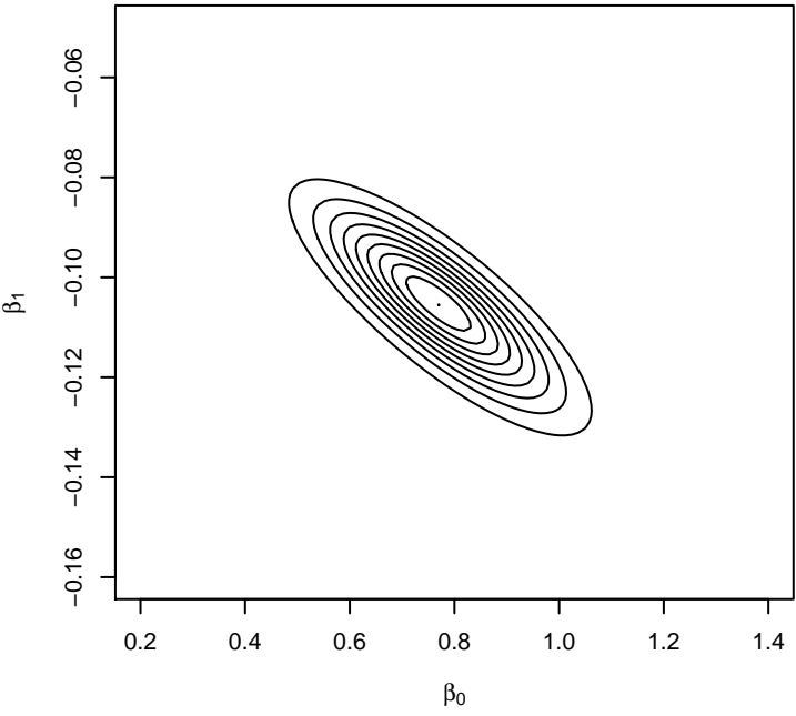
Posterior distribution
