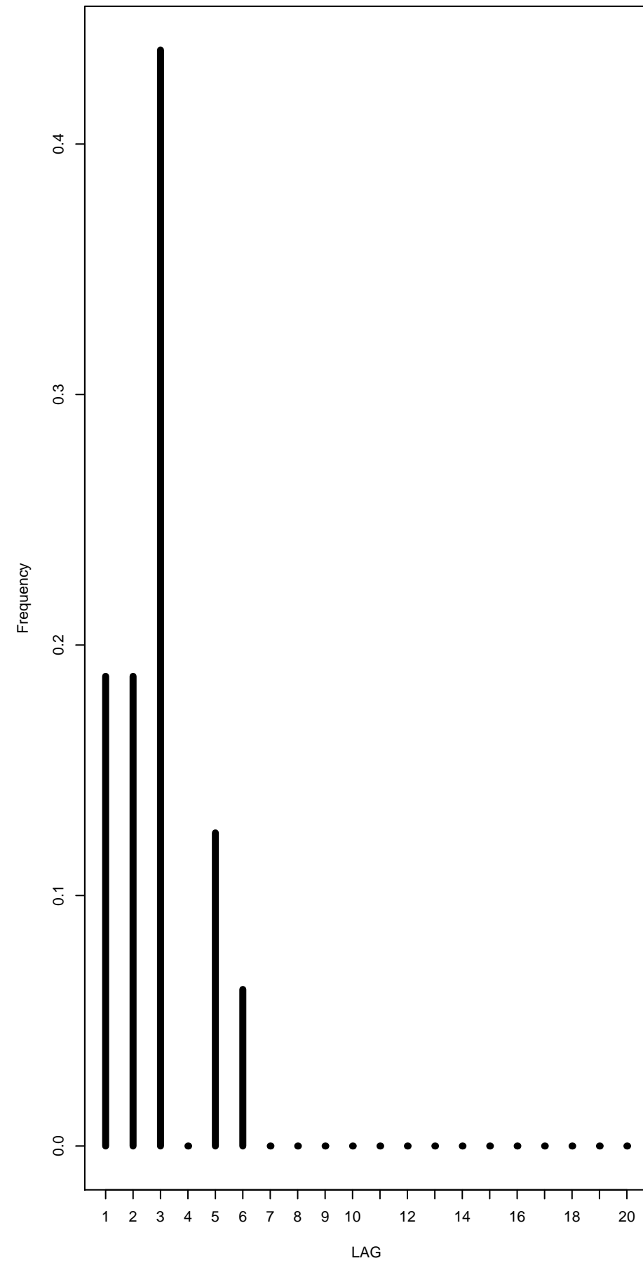
BIC n=120
